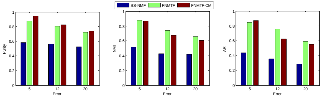
图 4 在不同聚类难度等级数据集下的四种指标对比结果( N=200 , K=5 )
