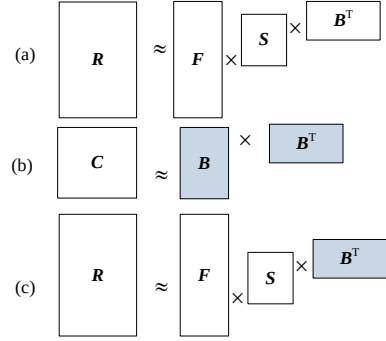
图 1 异构稀疏数据联合聚类框架
