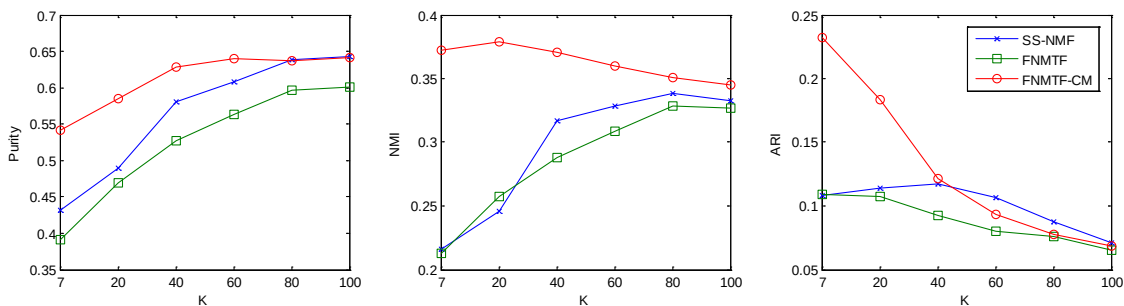
图 5 在 TITLE 数据集上不同聚类数目 K 的对比结果
