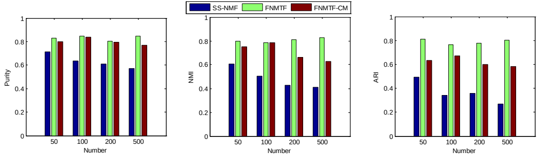
图 3 在不同节点规模 N 下的四种指标对比结果( K=5 , Error=12\% )
