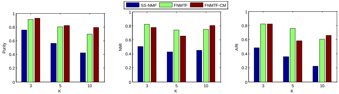
图 2 在不同聚类数 K 下的四种指标对比结果( N=200 , Error=12\% )
