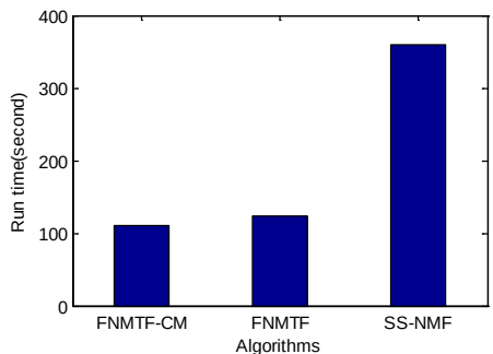
图 6 算法在 Weibo 数据集上的时间对比
